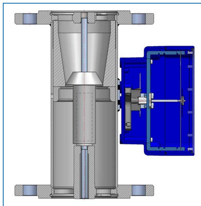
Tubo en EN 1.4404, PVC, PP o PTFE, en función de la versión de caudalímetro
